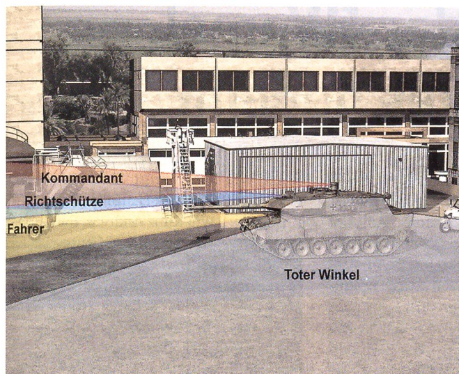
Die Grafik zeigt den für die Besatzung nicht einsehbaren Nahbereich durch die Winkelspiegel des Leopards. Der Fahrer sieht nur nach vorne, den Boden sieht er erst in zehn Metern Entfernung.
