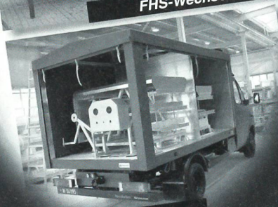
FHS-Spezial-Wechselaufbau
