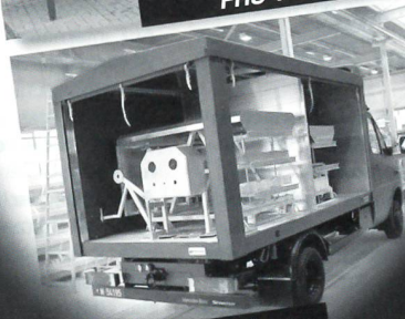
FHS-Spezial-Wechselaufbau
