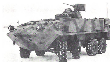
Radschützenpanzer
