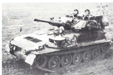
Spähpanzer Scorpion
