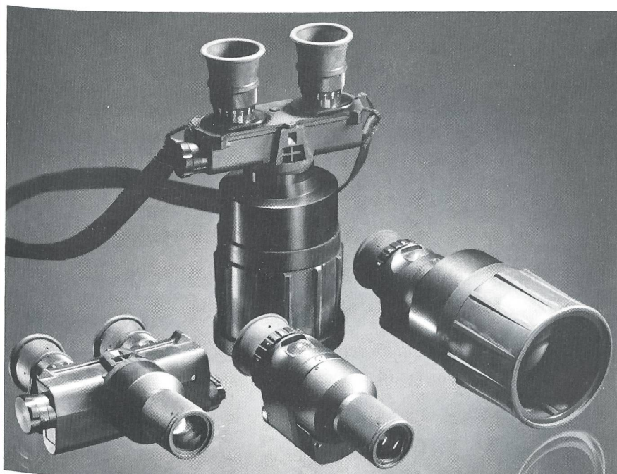
Die Restlichtverstärker-Gerätefamilie der Leica AG, Heerbrugg. – Vorne von links nach rechts: BIG25 Nachtsehbrille (hier ohne Kopfhalterung), BIM25 monokulares Nacht-Pocketscope (1×), BIM35 monokulares Nacht-Pocketscope (3×). Hinten, stehend: BIG35 handgehaltene Nachtfernglas (3×). Aus «Forum» Nr 12/93
