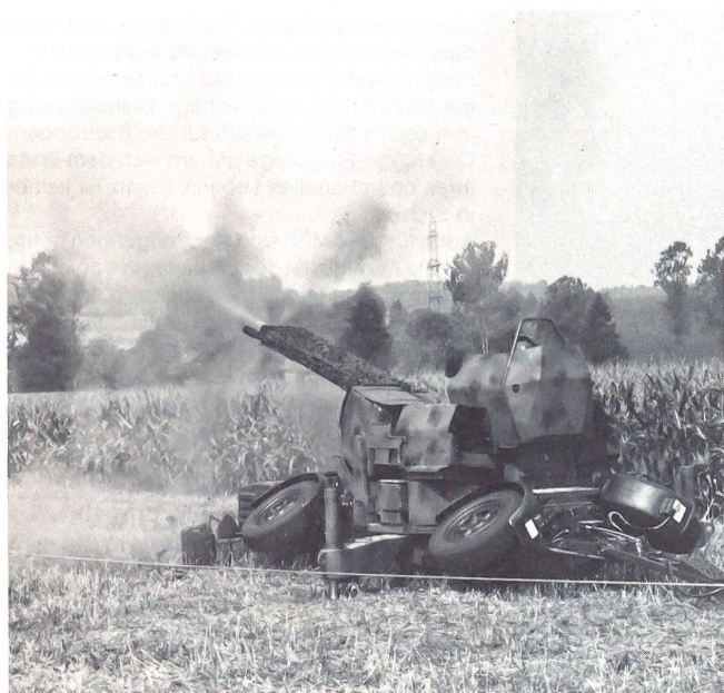
Den Gästen und der Presse wurde die kampfwertgesteigerte 35mm Flab Kan 63/90 im Einsatz «live» mit Zerfallmunition vordemonstriert.
