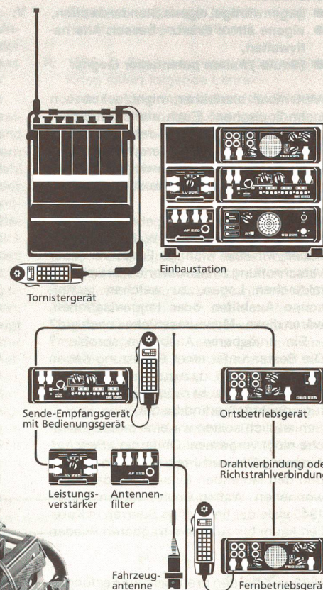
Das taktische Funksystem SE-225 TAMINA
