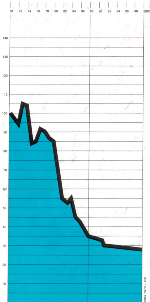
Schwefeldioxid
