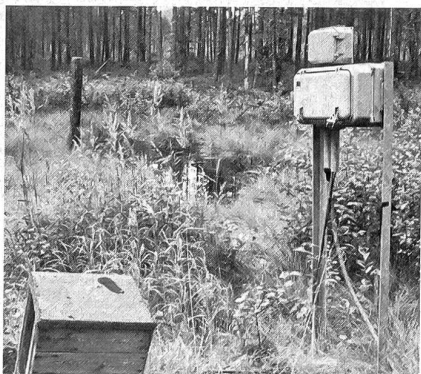
Zum Seismologischen Observatorium gehören auch eine Anzahl aussenstehender Stationen wie beispielsweise diese Schalldose für den kurzperiodischen Bohrloch-Erdbebenmesser.
