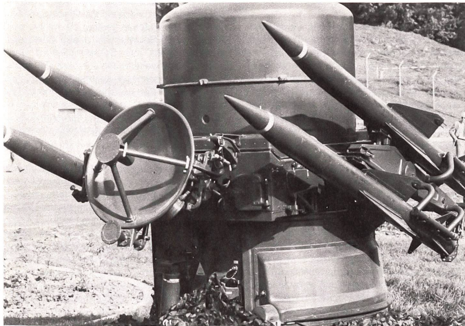
Der Lenkwaffenwerfer mit Suchradar (unter Radom), Gerät zur elektronischen Identifikation Freund-Feind (IFF), Kommandosender, Digitalrechner und vier Werferarmen zum Abschliessen von Kampflenkaffen
