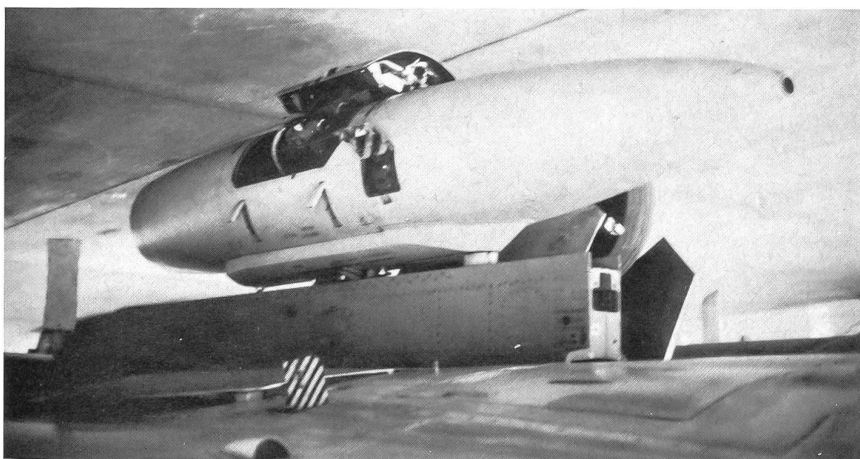
Die Mirage IIIRS des UeG können alle mit dem modernen Aufklärungsbehälter «Red Baron» der schwedischen Firma FFV ausgerüstet werden. Dieser Behälter beinhaltet das hochmoderne Zeilenabtastrgerät RS-730 von Texas Instruments, mit dem Infrarotaufnahmen bei Tag und Nacht gemacht werden können.
