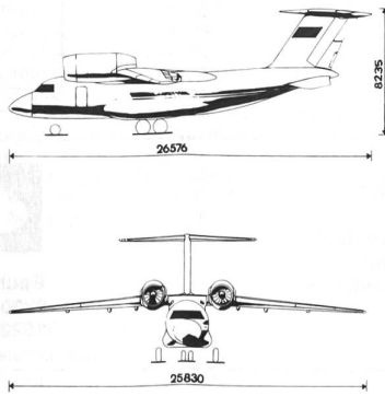
Antonov AN-72 NATO-Codennamen «Coaler» Taktischer STOL-Kampffronttransporter (ADLG Nr. 12/79) ka
