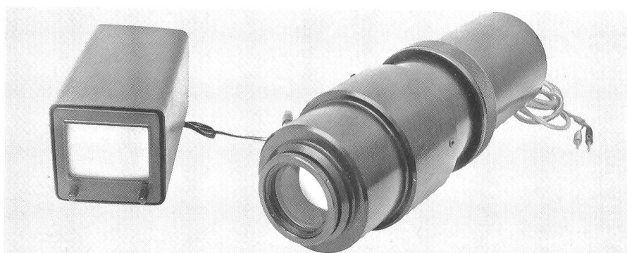
Restlichtverstärker-Kamera (LLL-TV)
