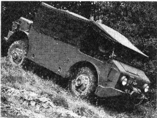
Geländegängiges Mannschafts- und Schleppfahrzeug der Artillerie, Typ 4MH, von Saurer-Berna, 1946.
