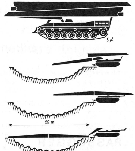
BRÜCKENPANZER «LEOPARD»
