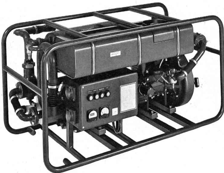
Generator-Pumpen-Aggregat für Wasseraufbereitungs-Anlagen
