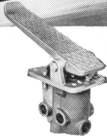
Zweikreis-Steuerventile BEKA
