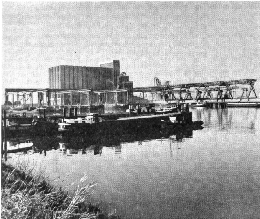
BÜHLER-Umschlags- und Siloanlage im Hafen Botlek (Rotterdam) Leistungen: Entladung = 1600 Tonnen pro Stunde, Beladung = 2800 Tonnen pro Stunde!
