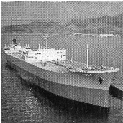
Der 69000-Tonnen-Motortanker «Ise Maru» wird von einem Ishikawajima-Harima-Sulzer-Zweitakt Dieselmotor, Typ 9 RD 90, angetrieben. Dieser neunzylindrige Hauptmotor von 900 mm Bohrung, 1550 mm Hub und 19800 PS Dauerleistung bei 119 U/min verleiht dem Tanker eine Geschwindigkeit von 15,5 Knoten.
