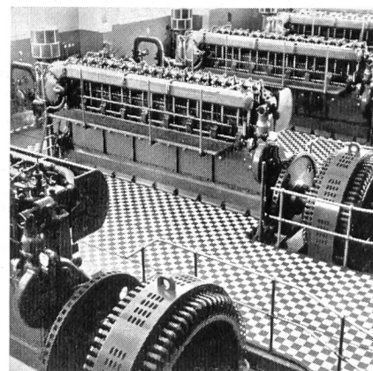
Im Rahmen des Bewässerungssystems von Bayara (Ägypten) sind Sulzer-Viertakt-Dieselmotoren eingesetzt. Sie entwickeln Leistungen von 3600 PS.
