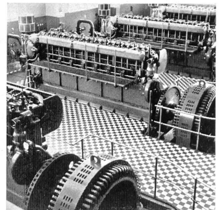
Im Rahmen des Bewässerungssystems von Bayara (Ägypten) sind Sulzer-Viertakt-Dieselmotoren eingesetzt. Sie entwickeln Leistungen von 3600 PS.
