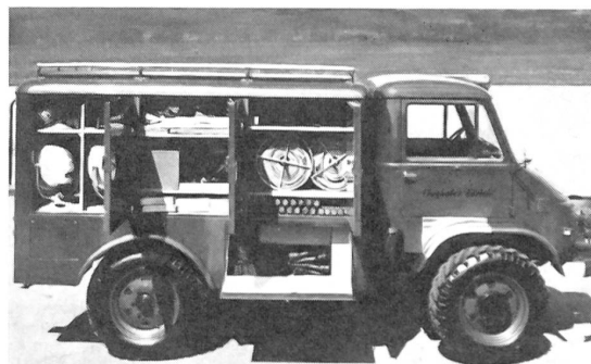
UNIMOG-S als Pionierfahrzeug
