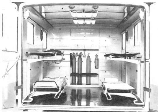
Krankentransportfahrzeug für 4 liegende oder 12 sitzende Patienten
