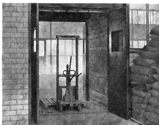
Beispiel: Etagen-Hebebühne
