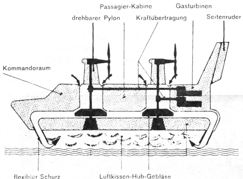
Prinzipschema eines Luftkissenfahrzeuges
