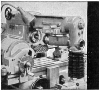
Maschine, ausgerüstet mit Universal-Teilapparat
