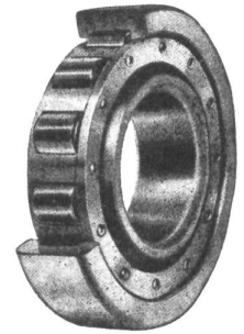
Rollenlager Präzisions-Stahlrollen
