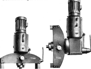
Typ HDE-TR Druckeinheiten
