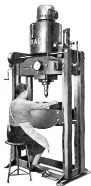
Typ JP-N Viersäulen- Jochpresse mit verstellbarem Arbeitstisch für Presskolben- drücke 0-25, 0-50, 0-100 Tonnen
