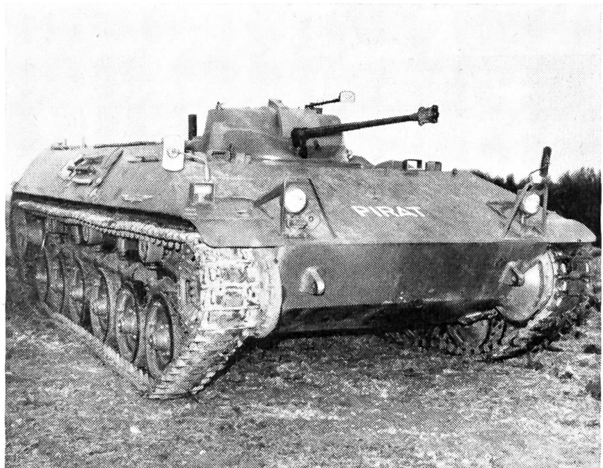
MOWAG Schützenpanzerwagen «PIRAT»
