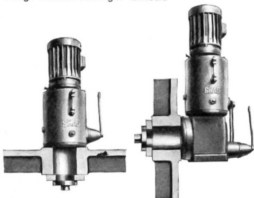
Typ HDE-TR Druckeinheiten
