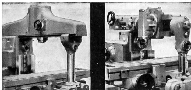
Oberarm «hvv» mit eingebauter Vertikalfrässpindel
