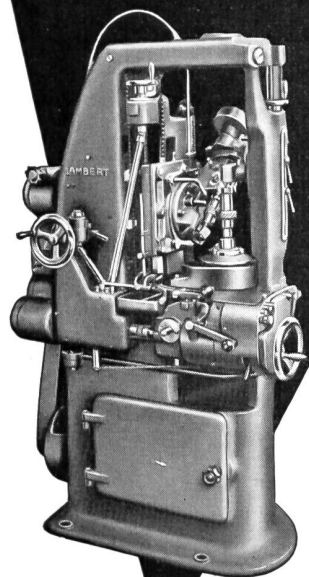
HALBAUTOMATISCHE UNIVERSAL-ABWÄLZ- RÄDERFRÄSMASCHINE
