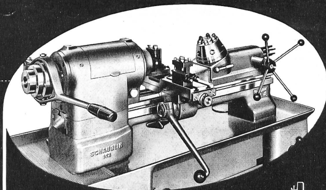
REVOLVERDREHBANK
