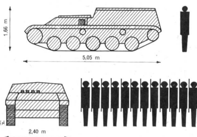
SCHÜTZENPANZERWAGEN MOWAG «PIRAT-SPW»
