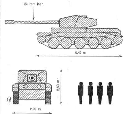
MITTELSCHWERER PANZER «CHARIOTEER»
