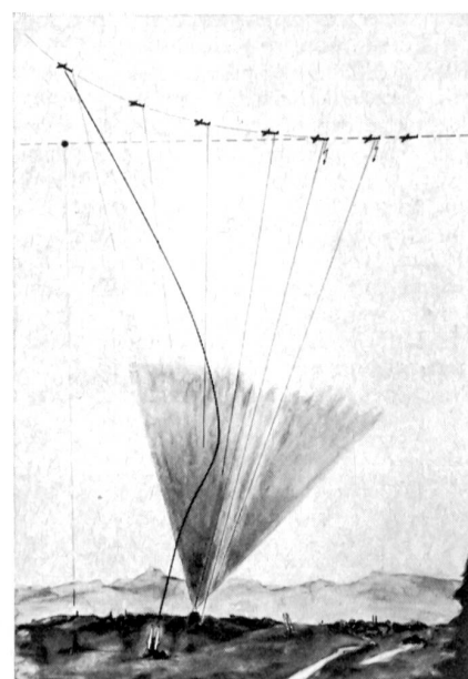
Leitstrahlenprinzip
