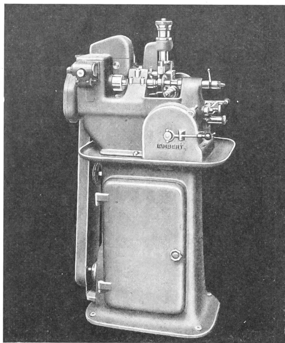
Abwälzräderfräsmaschine Type 75
