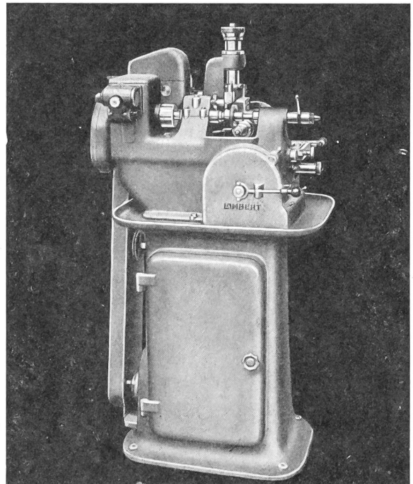
Abwälzraderfräsmaschine Type 75
