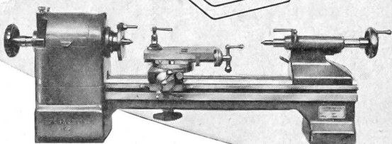
WERKZEUGMACHER-DREHBANK
