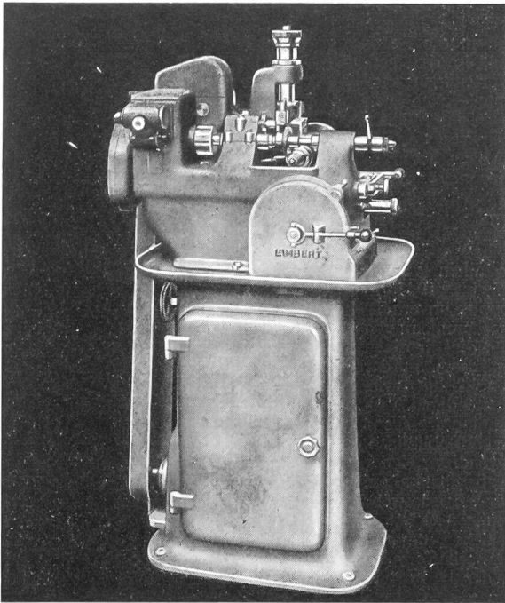
Abwärlzräderfräsmaschine Type 75
