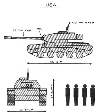
LEICHTER PANZER M.41 "WALKER BULLDOG"
