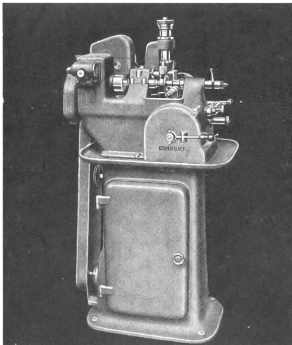
Abwälzräderfräsmaschine Type 75
