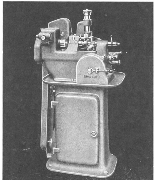
Abwälzraderfräsmaschine Type 75
