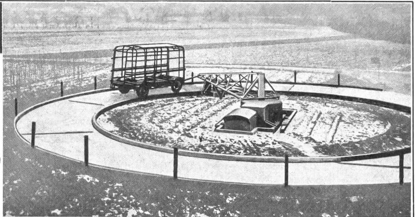
Lenksystem eines Anhängers wird auf werkeigener Versuchsbahn erprobt
