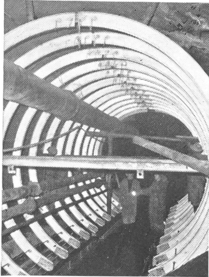
Druckstollen Dixence—Bagnes, 8500 m lang Lehrbogen für die Stollenschalung
