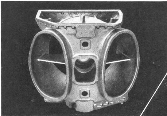
Gussstück für Ghost — Lizenz De Havilland
