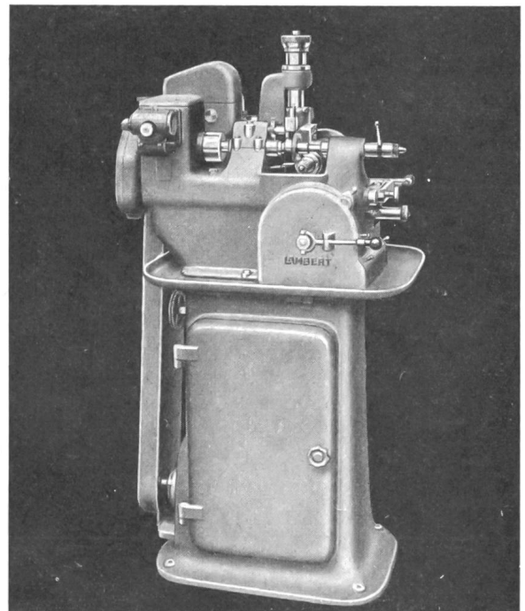
Abwälzräderfräsmaschine Type 75
