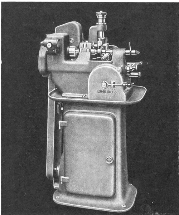
Abwälräderfräsmaschine Type 75
