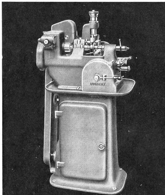
Abwälzräderfräsmaschine Type 75
