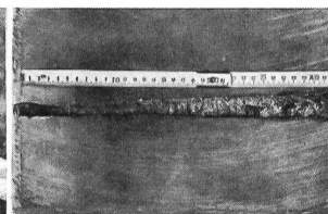
Wirkung der Hohlladung 8-cm-Panzerrakete
