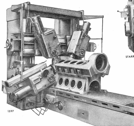
PORTAL Fräsmaschine Type P-1200 Tisch 3500×1200 mm
