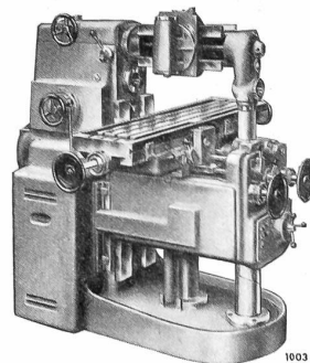
UNIVERSAL Fräsmaschine Type S-100 Tisch 1200×300 mm
