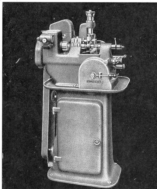
Abwälzraderfräsmaschine Type 75
