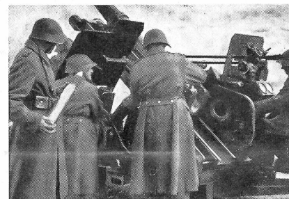
Eben ist eine 7,5-cm-Granate tempiert worden. Der Lader (Mitte) ist gerade im Begriff, sie aus dem Tempierstutzen zu ziehen, um sie anschließend zum Verschieben ins Patronenlager (rechts des Laders) zu schieben. Ganz rechts der Höhenrichter.
