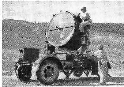
Schweizerischer Flab-Scheinwerfer.
